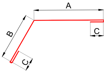
KEY: 3 - Lemovacia lišta
