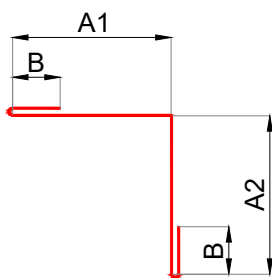
KEY: 4 - Lemovacia lišta
