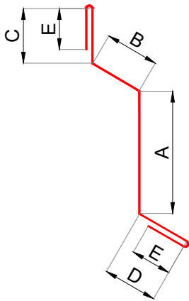
KEY: 2 - Soklová odkvapnica
